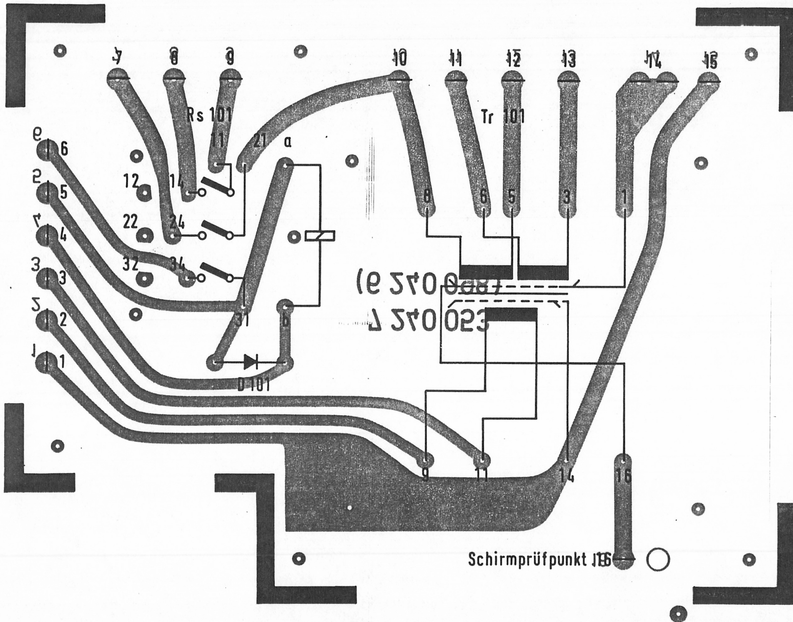
Sicht auf Bauelemente-Seite View of component side
