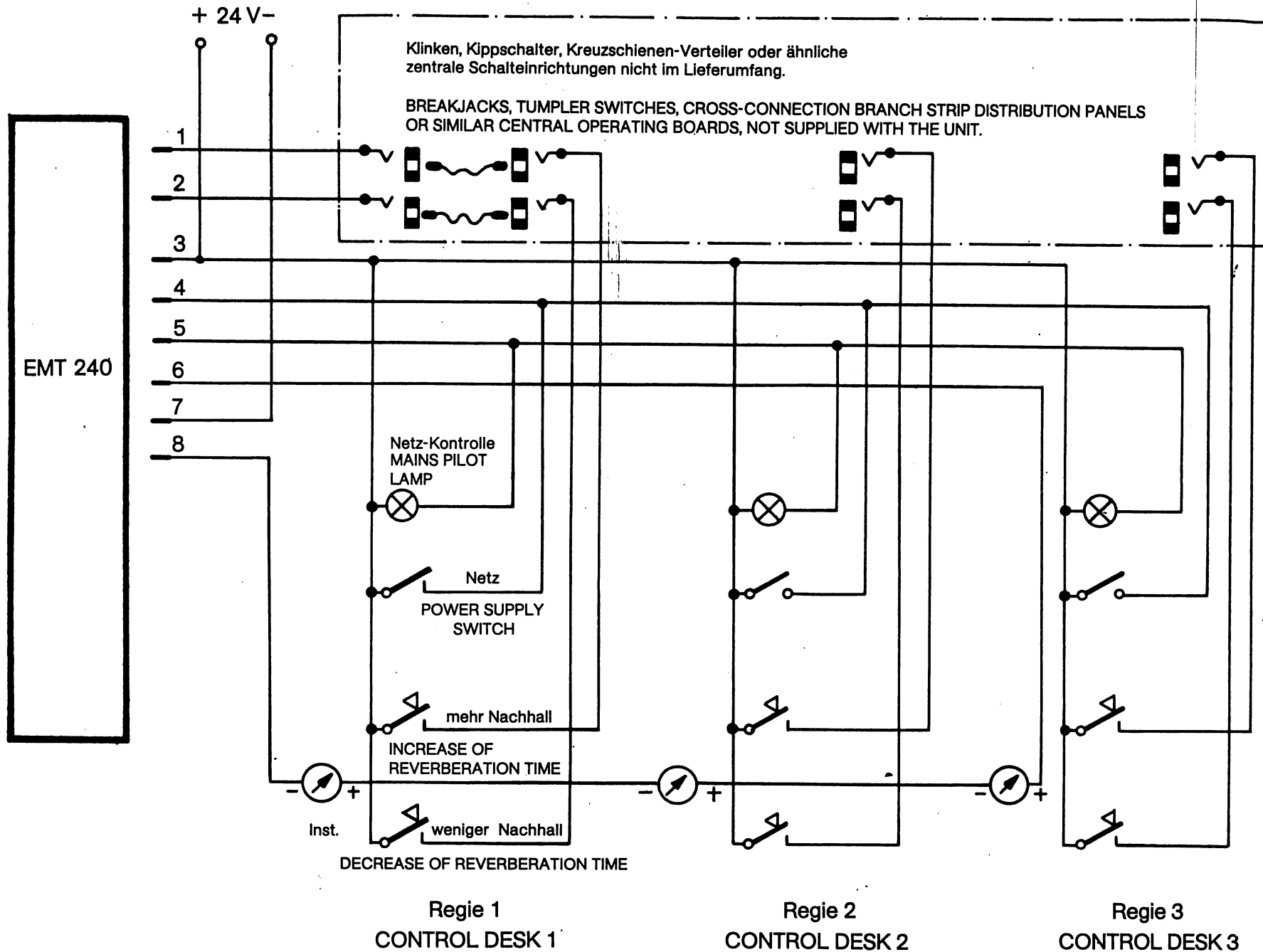
Schaltung mehrerer Regie-Bedienungsteile Circuit diagram for multiple control desk arrangements EMT 240
