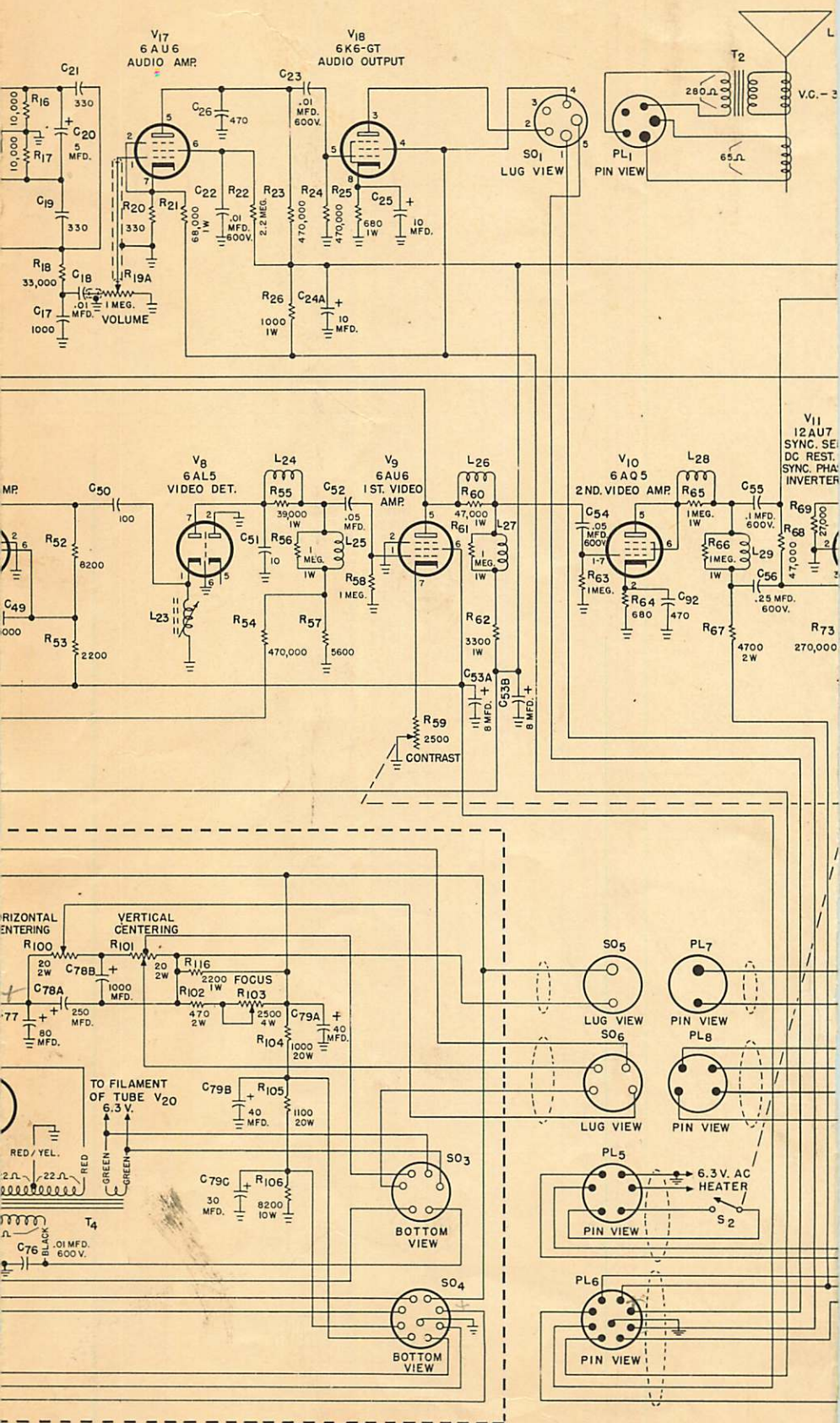
Fig. 18. Schema
